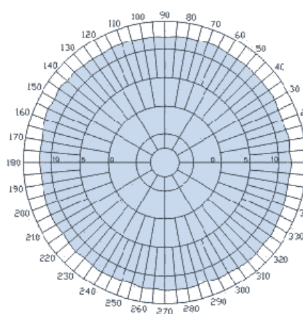
H-Plane
