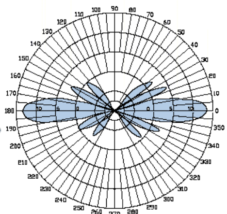
E-Plane
