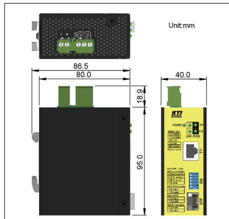
Din-Rail Mount Dimensionn
