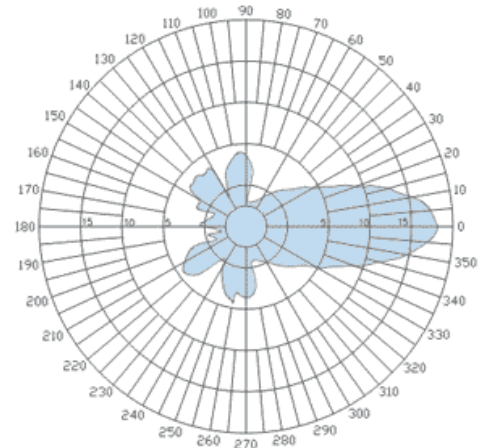
E-Plane
