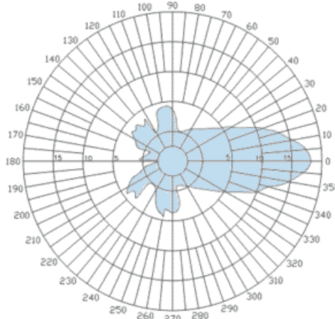
H-Plane
