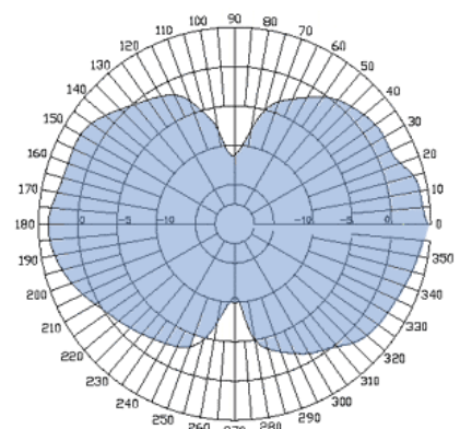
E-Plane
